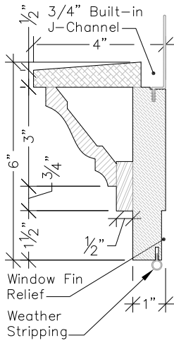
Section A-A 3"=1'-0"
