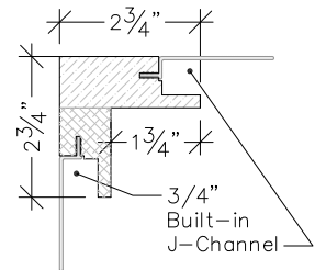
Section A-A 3"=1'-0"
