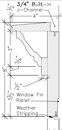
Section A-A 3"=1'-0"
