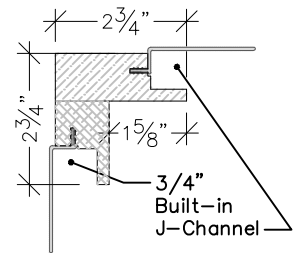
Section A-A 3"=1'-0"
